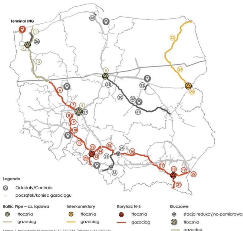
Rysunek 9. Inwestycje kluczowe realizowane w 2018 roku przez OGP Gaz-System S.A.
